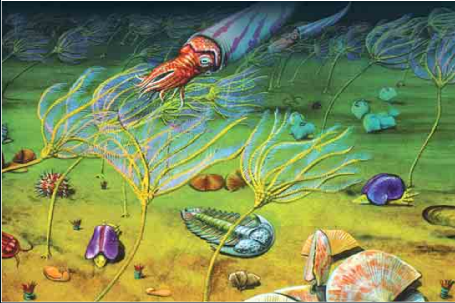
Kambriyen döneminde yaşamış olan canlıları gösteren temsili bir resim
