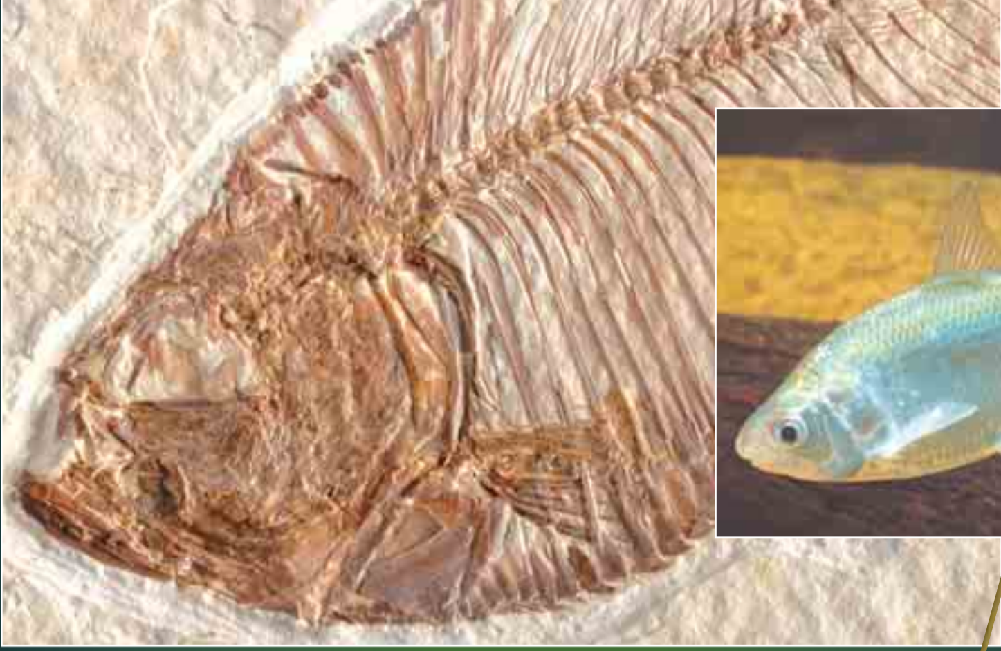
48 - 37 milyon yıllık ringa balığı fosili
