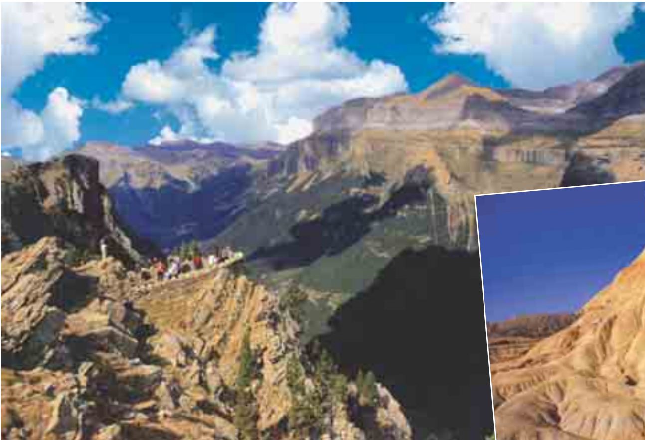
600 metre yüksekliğindeki kireçtaşı kayalarından oluşan Ordesa kanyonu.
