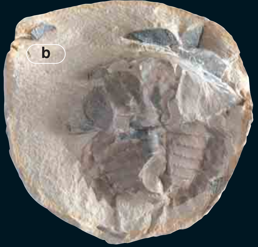
Resimde görülen fosil, negatif - pozitif görümlü çift parçalı bir fosildir.
